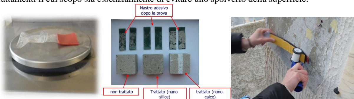
Figura: (a) nastro adesivo tagliato sul piatto della bilancia; (b) esempio di risultato ottenibile dalla prova; (c) test in situ presso la Torre intitolata ai caduti del secondo conflitto mondiale (Torricella Peligna, CH)
